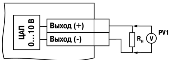
Рисунок Б.8 – Схема подключения нагрузки к ВЭ типа «У». R_n > 2 \text{ кОм}
