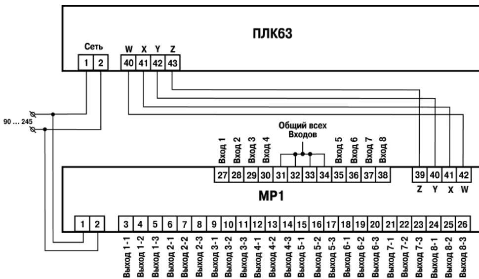
Рисунок Б.14 – Схема подключения модуля MP1 к ПЛК63
