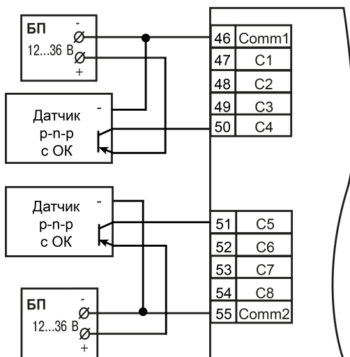
Рисунок Б.2 – Схема подключения р-п-р датчиков
