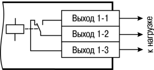
Рисунок Б.13 – Схема подключения нагрузки к ВЭ типа «Р» (для первого ВЭ)
